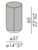
tavolo basso - low table TB-35R METAL
