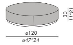
tavolo basso - low table TB-120R METAL
